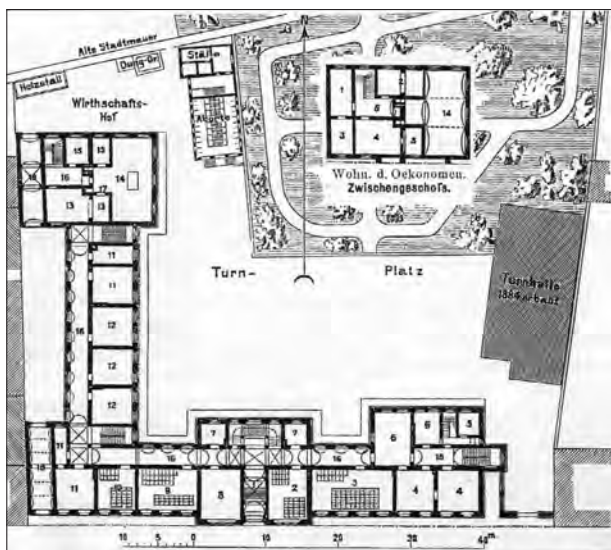
Abb. 14: Grundriss des Erdgeschosses. Zentralblatt der Bauverwaltung IX (1889). Aus: Hussong: Lorenz-Kellner-Schule (Anm. 72), S. 354.
