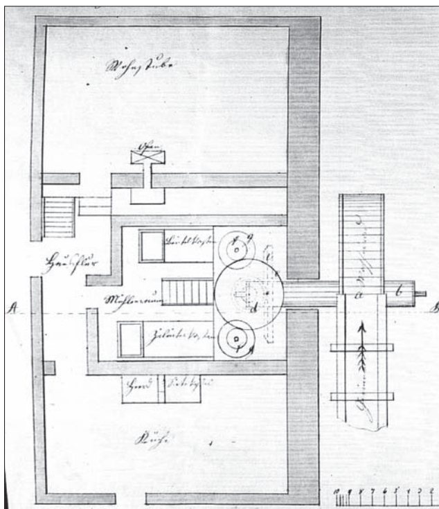
Abb. 7: Grundriss der Beekmühle, 1860. Quelle: ThStAG: Kreisausschuss Heiligenstadt, 982, Bl. 6.
