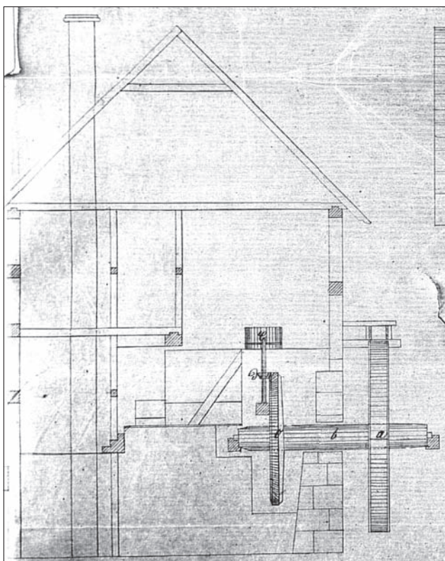
Abb. 9: Schnitt durch die Obermühle, 1863. Quelle: ThStAG: Kreisausschuss Heiligenstadt, 983, Bl. 8.
