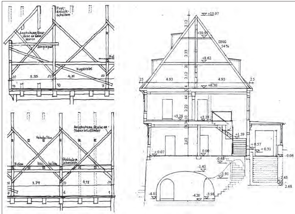
Abb. 16: Links oben: Längsschnitt der Dachkonstruktion mit Firstständergerüst Achse 1–7, angepasster Zustand von 1599. Links unten: Längsschnitt der Dachkonstruktion wie links oben, Achse 7–13 Zustand 1437. Rechts: Gebäudequerschnitt mit Höhen der Einzelgeschosse. Zeichnung: K. A. Heidenblut.
