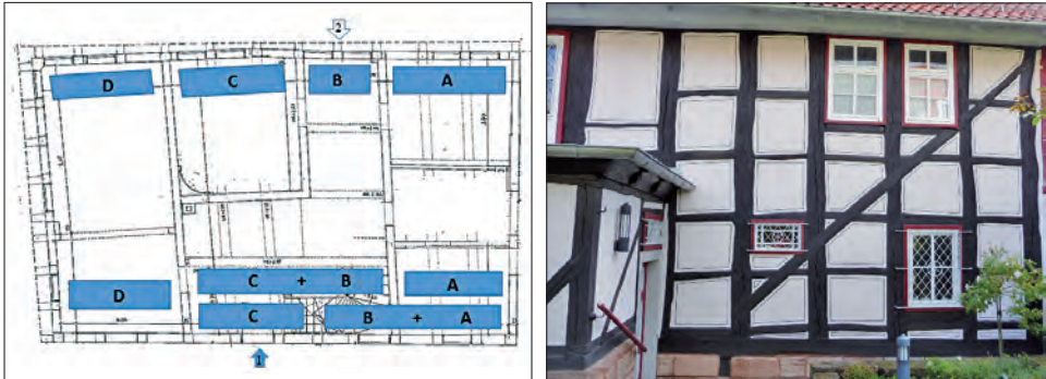
Abb. 7: Links: vierzoniger Schemagrundriss des 1. Stockwerkes, (1) traufseitiger Eingang in die Westfassade, (2) zwischenzeitlicher traufseitiger Eingang in die Ostfassade (1840–1935); rechts: Detail der zweigeschossigen Ständerfassade auf der Hofseite mit Verstrebung über vier Felder und zwei Stockwerke. Zeichnung/Foto: K. A. Heidenblut.
