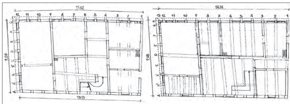
Abb. 8: Links: Grundriss des 1. Stockwerks, rechts Grundriss des 2. Stockwerks mit Maß- und Achsangaben. Zeichnung: K. A. Heidenblut.
