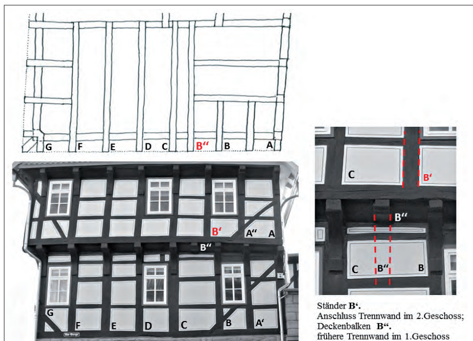
Abb. 14: Nordgiebel und Konstruktionslösung der Giebeleckräume. Oben: Deckenbalkenlage des ersten Stockwerks. Unten: Fachwerk des Nordgiebels. Rechts: Detailausschnitt mit Darstellung der ursprünglichen Wandanschlüsse im ersten Stockwerk (B') und zweiten Stockwerk (B'). Foto/Zeichnung: K. A. Heidenblut.
