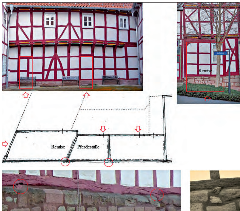
Abb. 17: Oben links: Westfassade des Marstalls mit Eingängen zu den Pferdeställen. Oben rechts: Südgiebel mit früherer Toreinfahrt zur Remise. Mitte: Grundriss des Marstalls. Unten: Schwelkenköpfe für die Schottenwände in Ställen unter der Schwelle der Fachwerkfassade. Fotos/Zeichnung: K. A. Heidenblut.
