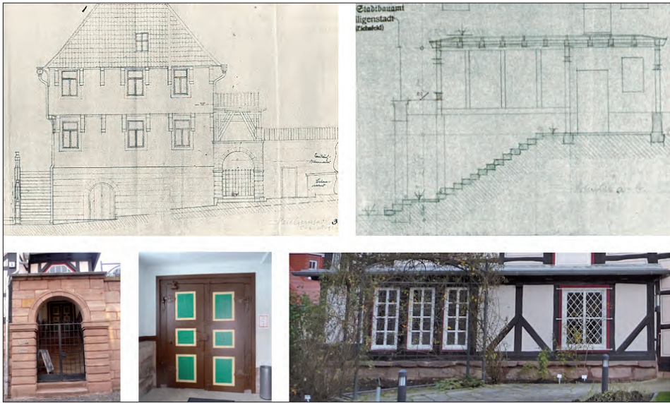
Abb. 25: Eingangsbauwerk von 1935 als Anbau an die Westfassade. Oben links: Nordansicht. Oben rechts: Längsschnitt. Planung des Stadtbauamtes zum Bau des neuen Eingangs an der Westseite. StadtA HIG. Unten von links: Portal des Eingangsbauwerks, aus der Ostfassade umgesetzte neobarocke Tür, Gartenansicht des Eingangsbauwerks. Fotos: K. A. Heidenblut.
