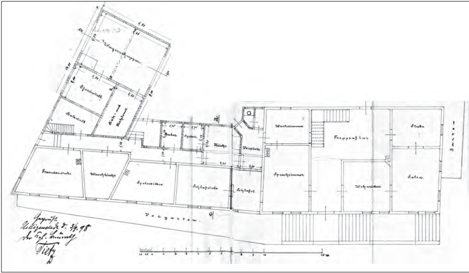
Abb. 22: StadtA HIG: Martinsches Haus. Planung für den Umbau im ersten Stockwerk, 1898.
